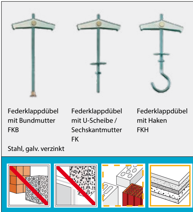
FKB - mit Gewindestange und Bundmutter
